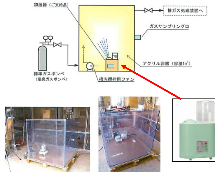
試験装置概略図
